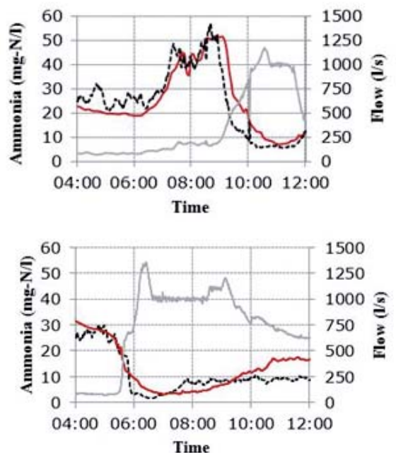
Figur 5 Målt og beregnet ammonium koncentration.
