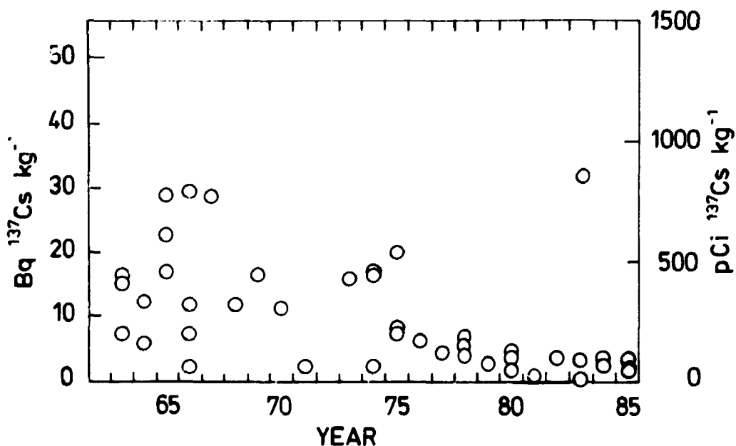
Fig. 2.2.7.4.1. Cesium-137 in Faroese potatoes, 1962-1985.
