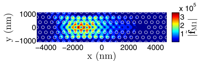
(d) Disordered ( \sigma_{Dis} = 0.04a ) cavity mode profile, f_3 above
