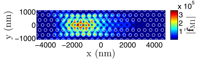
(d) Disordered ( \sigma_{\text{Dis}} = 0.04a ) cavity mode profile, f_3 above
