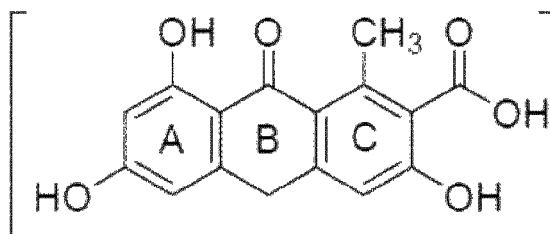
FK antrone
