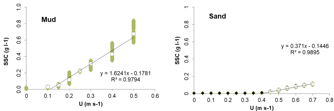
Figur 4.2. viser resultaterne af erosionsforsøgene for sandet sediment (LOI=0.3%) og det mudrede sediment (LOI= 16.2%) gennemført i kontrollerede flumeforsøg med variabel strømhastighed ("U"). Erosionsmængden er angivet som koncentrationen af suspenderet stof (SPM).
