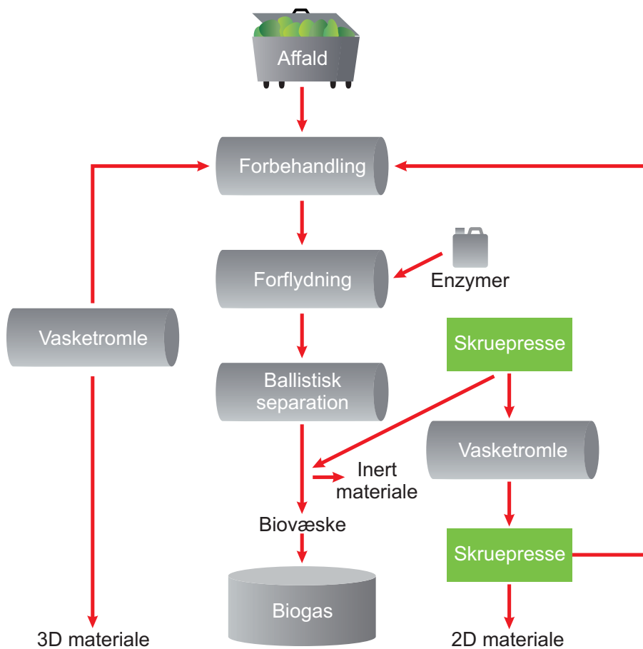
Figur 1 Princippet i Renaissance-teknologien
