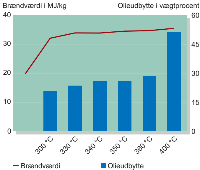
Udbytte og brændværdi for HTL-bioolie fremstillet af DDGS ved forskellige temperaturer.
