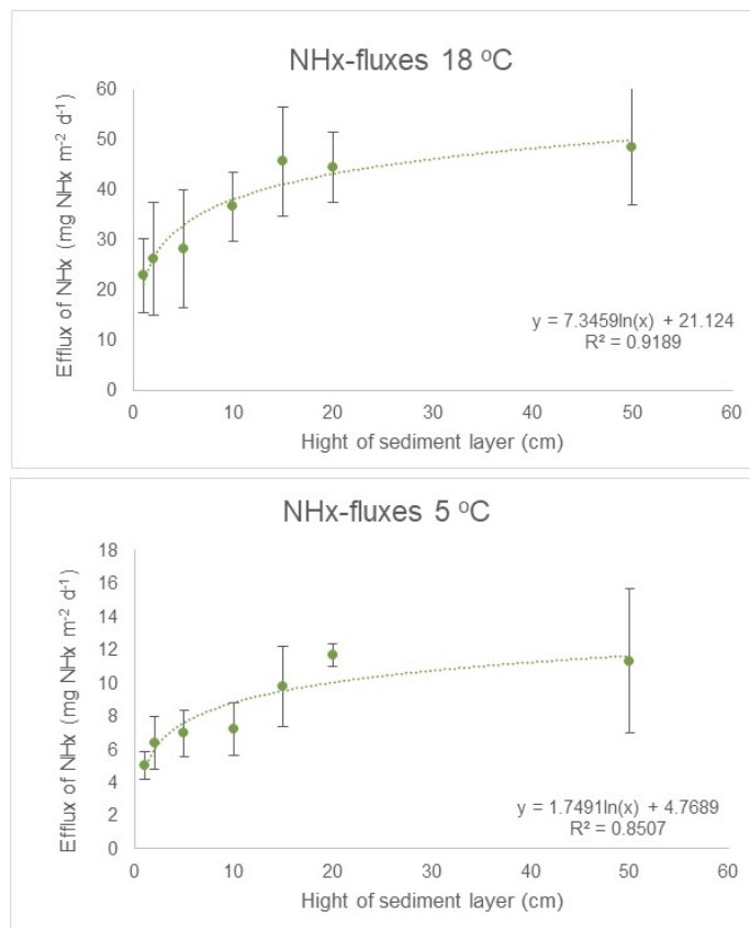
Figur 4.5. Figuren viser NH 4 -effluxens afhængighed af sedimentkernerens højde (x-akse på begge grafer) og temperatur, som i den øverste graf er 18 °C og nederst er 5 °C (upublicerede data, Flindt & Canal-Verges).
