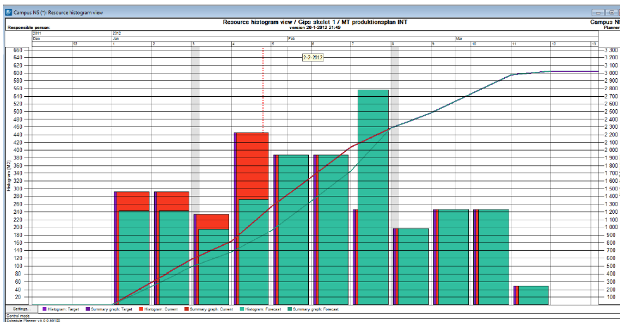
Fig. 4: Illustrationen viser et histogram beskrivende byggeriets stade og fremdrift. Histogrammet er knyttet til den digitale styringsmodel.
