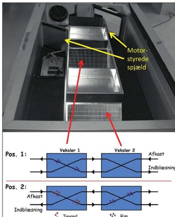
Figur 3. Billede og principskitse af varmeveksleren, der viser de to sammenkoblede vekslerunits og spjældet, der styrer hvilken unit, der kommer først i luftstrømmens retning.
