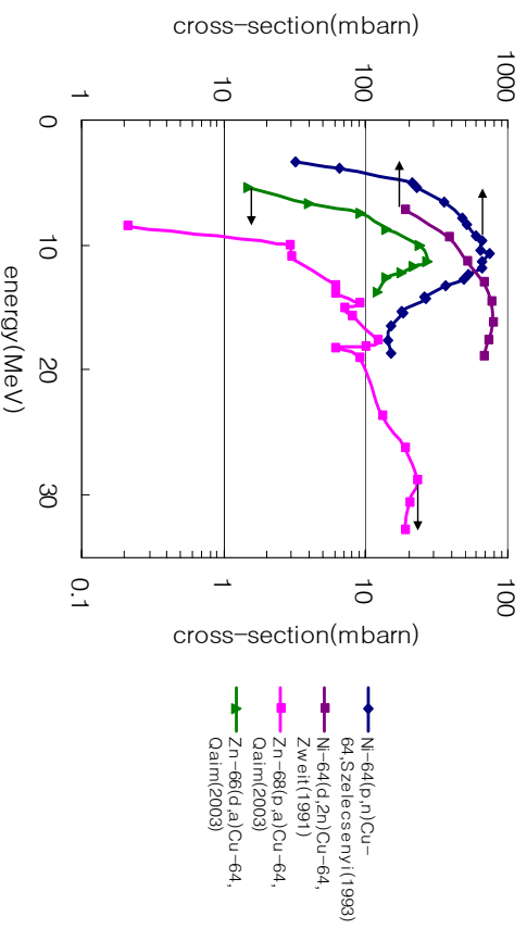
Fig. Excitation functions of ^{64}\text{Ni}(p,n)^{64}\text{Cu} and ^{64}\text{Ni}(d,2n)^{64}\text{Cu} , ^{68}\text{Zn}(p,\alpha)^{64}\text{Cu} , ^{68}\text{Zn}(d,\alpha)^{64}\text{Cu} . From Szelecsenyi, Zweit, Qaim
