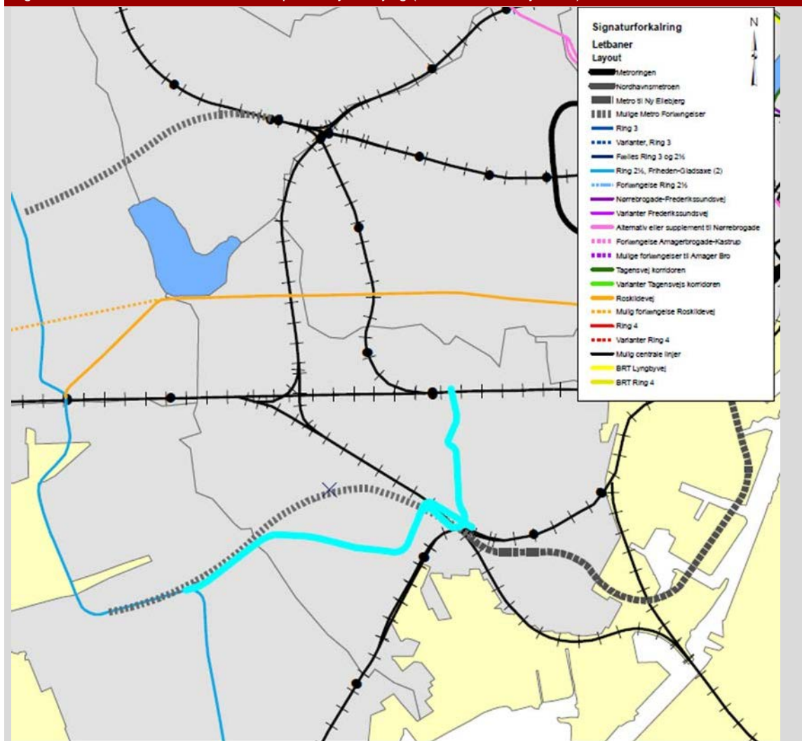
Figur C-14 Letbaneversion Hvidovre Hospital – Ny Ellebjerg (frømhævet med lyseblåt).
