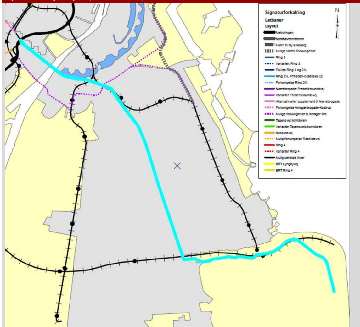
Figur C-16 Amagerbrogade (fremhævet med lyseblåt).
