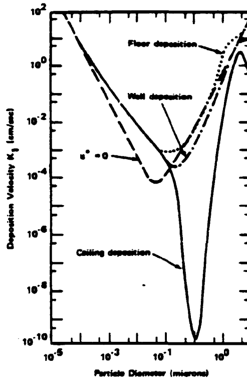
Fig. 4. Sammenligning af depositions- hastigheder til glatte overflader (gulv, væg og loft). U_* = 34,1 cm/s. Fra Sehmel (73)
