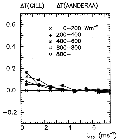
Fig. 7. Middel-forskellen mellem temperaturgradienten (9-2 m o.t.) bestemt med Gill skærm og Aanderaa skærm som funktion af den kortbølgede indstråling og vindhastigheden i 10 m. Risø, oktober 1985 - juni 1986.
