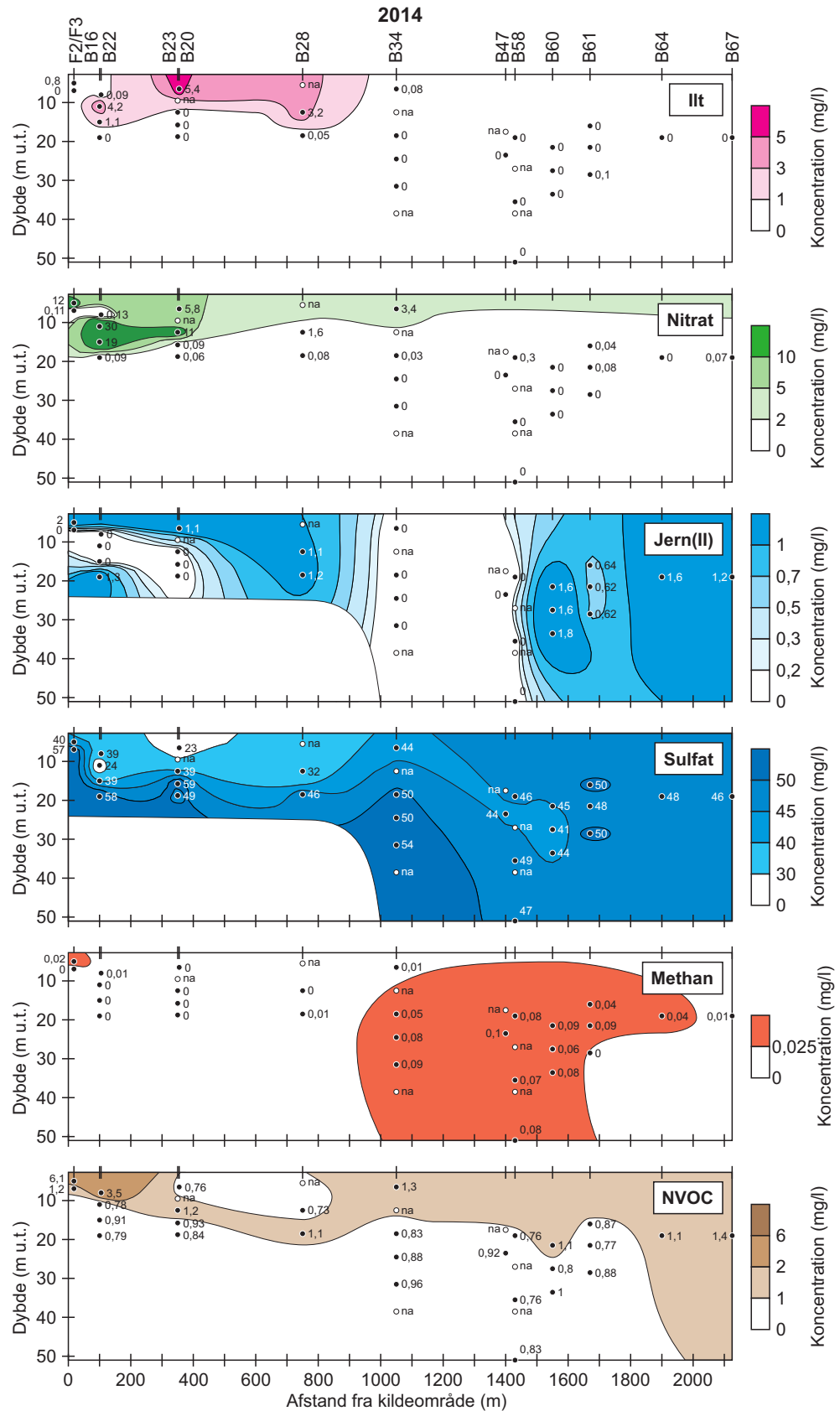
Figur 3.4b: Indhold af ilt, nitrat, opløst jern, sulfat og methan samt NVOC i grundvand (mg/L) i langsgående transekt 2014.
