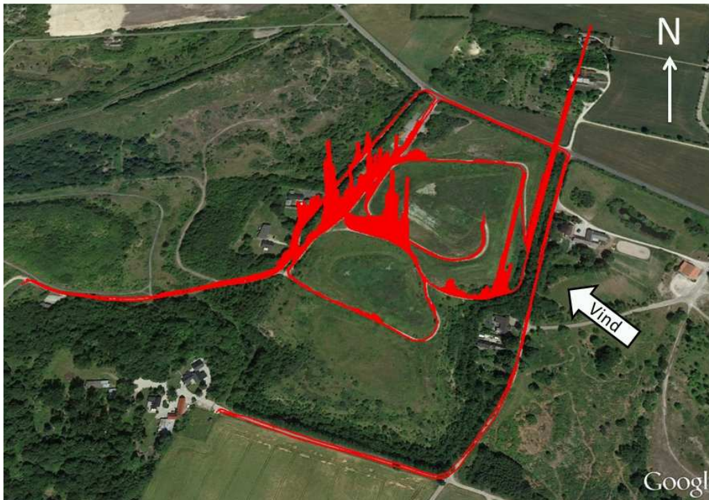
Figur 4. Metanscreening med fintfølede måleudstyr rundt på farbare veje på Hedeland deponi. Baggrundskoncentrationen af metan på 1920 ppb er fratrukket. Den højest målte metankoncentration er 6000 ppb over baggrund.
