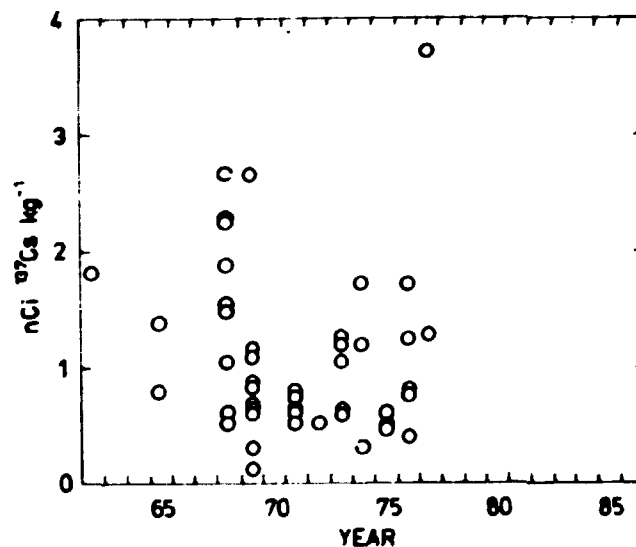
Fig. 2.3.1. Cesium-137 in mutton, 1962-1977.
