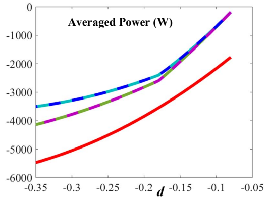
Fig. 7 (f) V_2 \rightarrow V_1 , V_1=601\text{V} , V_2=60\text{V} , N=15/3
