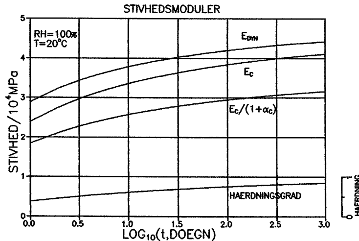
Figure 1 – Eksempel 1: Dyn. E-modul: E_{DYN} . Stat. E-modul: E_c . Modul for spontan + forsinket elastisk deformation, E_c/(1 + \alpha_c) . Hærdningsgraden er g .
