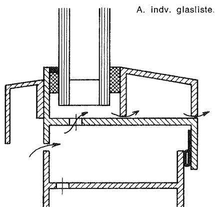
Fig. 11. Eksempel på metalbundramme med drænet glasfals.
