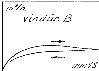
Fig. 3. Vindtætheden viser hysteres.
