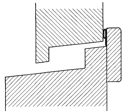
Fig. 10. Eksempel på bundfuge med 2-trins tætning.
