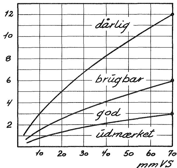
Fig. 8. Forslag til klassificering af vinduer efter vindtæthed pr. meter fuge.
