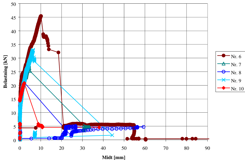
Figur 11. Kraftmålinger.
