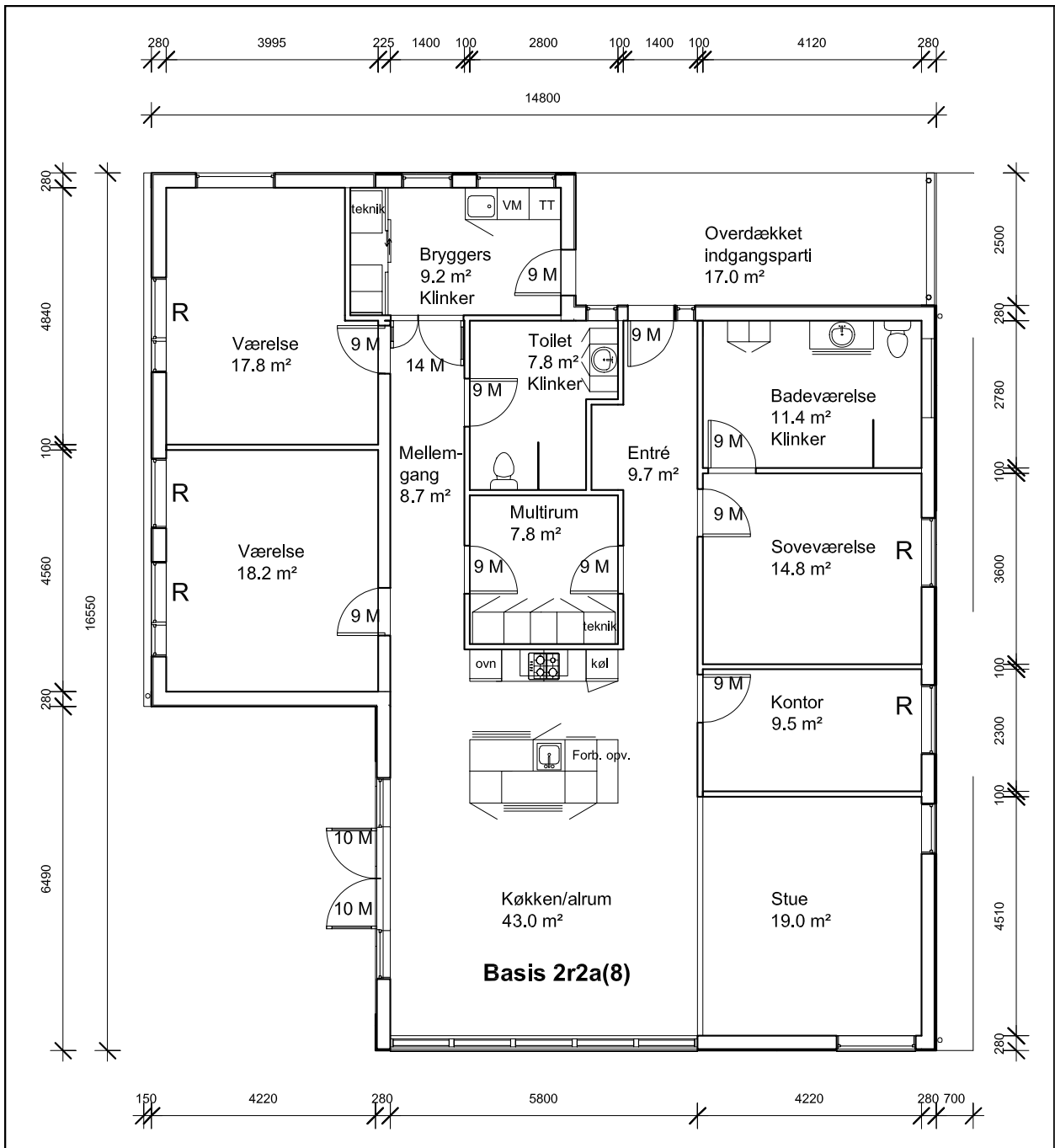
Figur 17. Plantegning.
