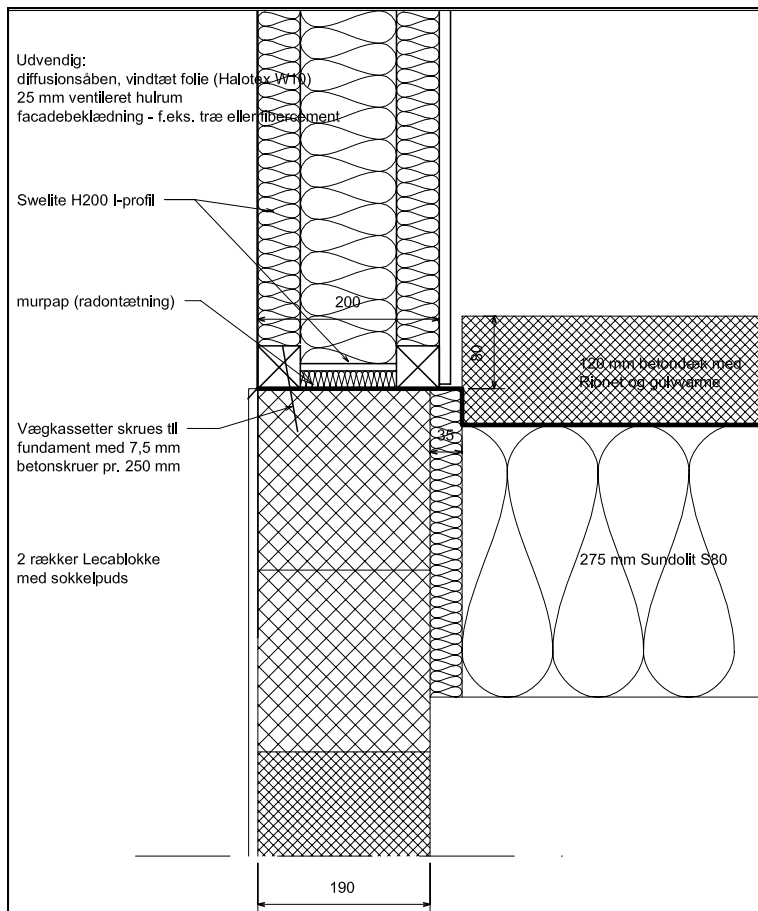
Figur 20. Samling mellem terrændæk og ydervæg.
