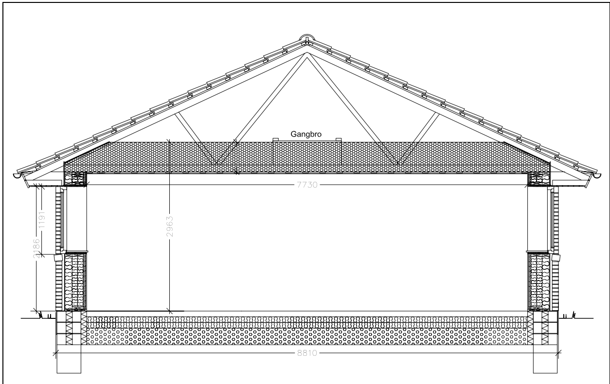
Figur 11. Tværsnit
