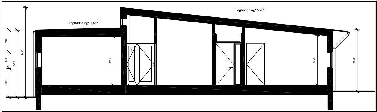
Figur 18. Tværsnit
