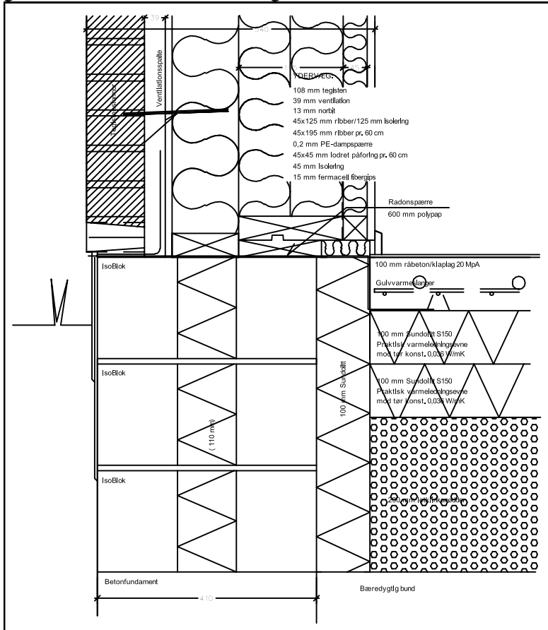
Figur 13. Samling mellem terrændæk og ydervæg.
