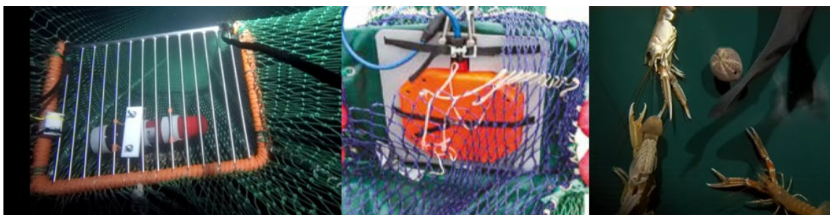
Figur 2. Fiskeriets CO 2 -udledninger kan reduceres ved brug af sensorer til realtidsmonitoring og -optimering af redskabsfunktion (venstre, midten) og ved brug af undervandskameraer til realtidsmonitoring af fangstsammensætning og optimering af fiskeriindsats (f.eks. ved at stoppe fiskeri eller skifte fangstplads når fangstrater er lave).
