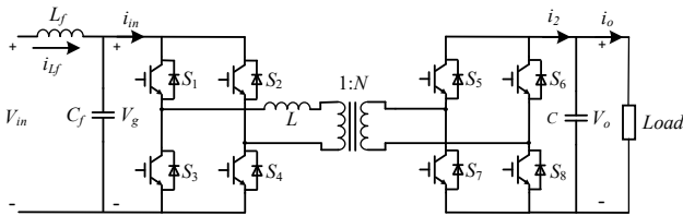
Fig. 1. DC-DC DAB converter.
