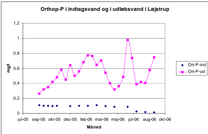
Figur 12 Orthofosfat-fosfor koncentrationen (mg/l) i indtagvandet og i udløbet til Hadsten Lilleå i det første måleår på Løjstrup Dambrug (øst).
