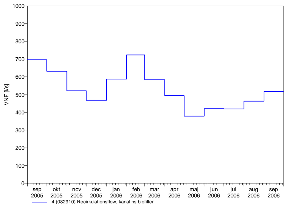
Figur 6 Recirkulationsflow, månedsmiddel l/s i Løjstrup Dambrug (øst), 1.måleår.
