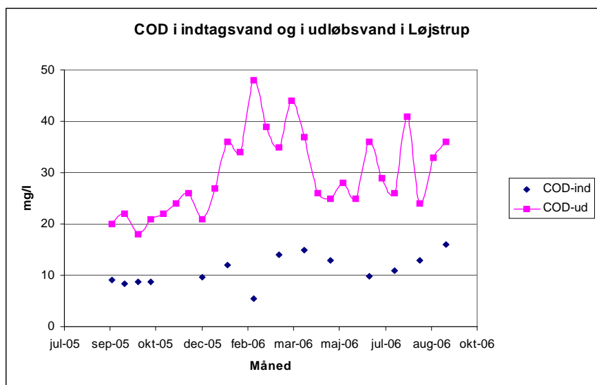
Figur 15 Organisk stof målt som COD koncentrationen (mg/l) i indtagsvandet og i udløbet til Hadsten Lilleå i det første måleår på Løjstrup Dambrug (øst).
