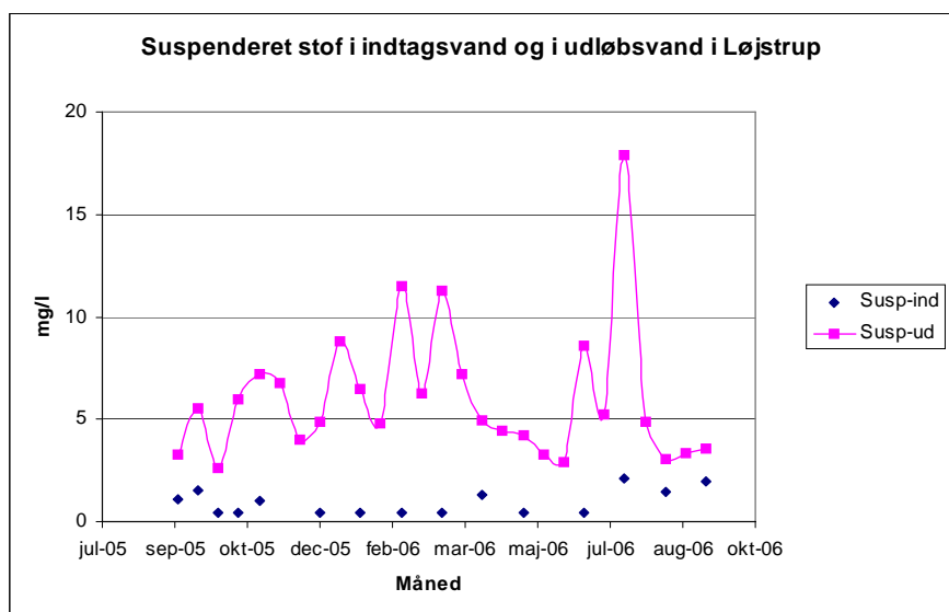
Figur 16 Suspenderet stof koncentrationen (mg/l) i indtagsvandet og i udløbet til Hadsten Lilleå i det første måleår på Løjstrup Dambrug (øst).
