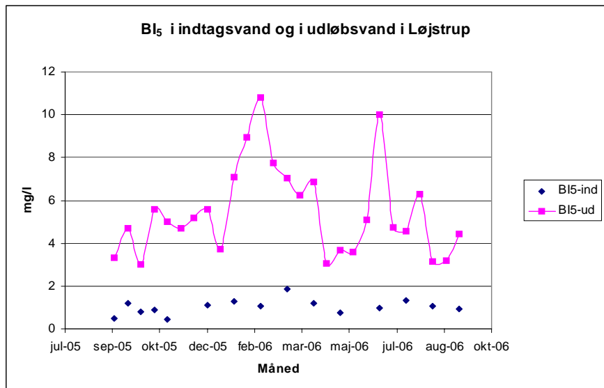
Figur 14 Organisk stof målt som BI 5 koncentrationen (mg/l) i indtagsvandet og i udløbet til Hadsten Lilleå i det første måleår på Løjstrup Dambrug (øst).
