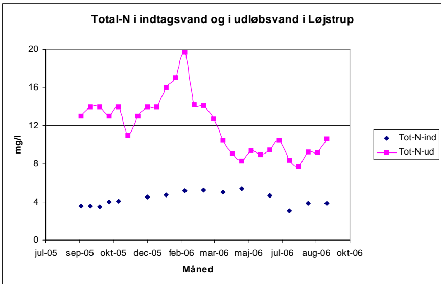
Figur 11 Total-kvælstof koncentrationen (mg/l) i indtagvandet og i udløbet til Hadsten Lilleå i det første måleår på Løjstrup Dambrug (øst).
