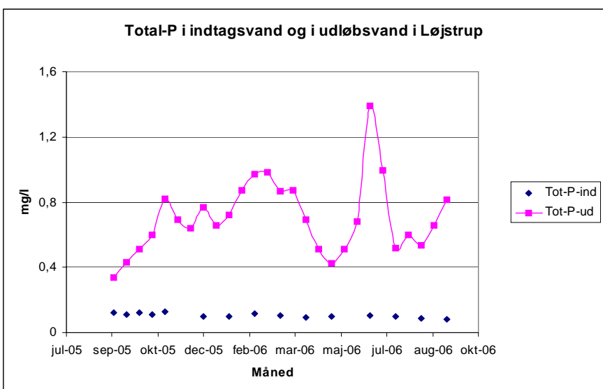
Figur 13 Total-fosfor koncentrationen (mg/l) i indtagvandet og i udløbet til Hadsten Lilleå i det første måleår på Løjstrup Dambrug (øst).
