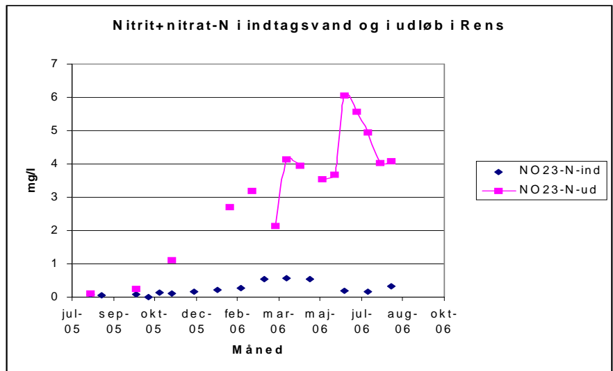
Figur 12 Nitrat+nitrit-kvælstof koncentrationen (mg/l) i indtagstvånd og i udløbet til Sønderå i det første måleår på Rens Dambrug.
