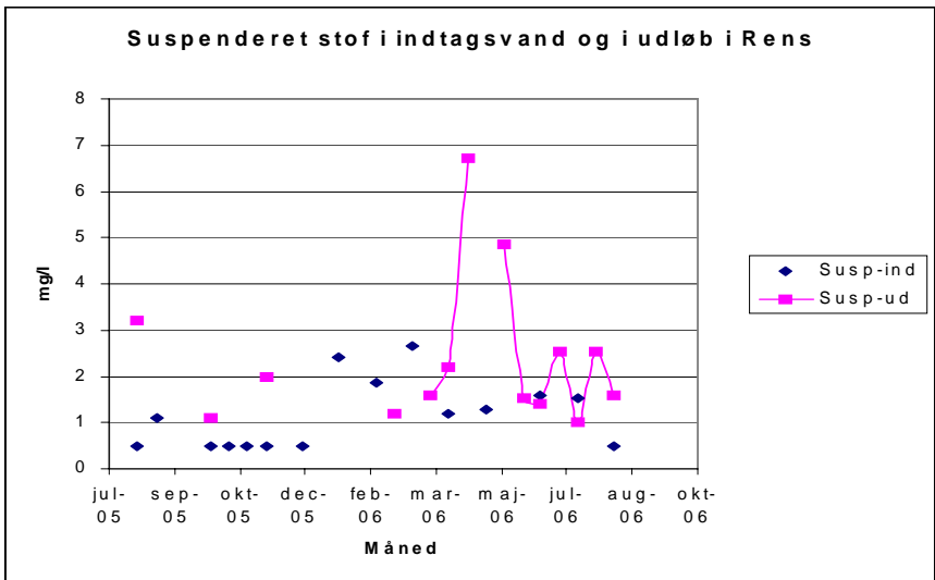
Figur 18 Suspendert stof koncentrationen (mg/l) i indtagsvandet og i udløbet til Sønderå i det første måleår på Rens Dambrug.
