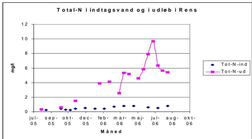
Figur 13 Total-kvælstof koncentrationen (mg/l) i indtagstvåndet og i udløbet til Sønder Å i det første måleår på Rens Dambrug.
