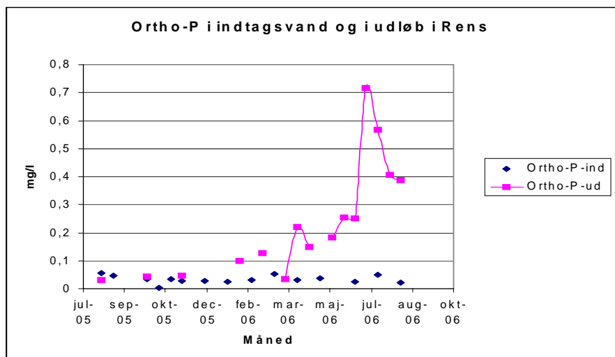
Figur 14 Orthofosfat fosfor koncentrationen (mg/l) i indtagstvåndet og i udløbet til Sønderå i det første måleår på Rens Dambrug.
