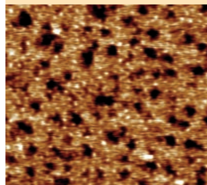
Nogle typer plaster bliver til ved, at man tilsætter en olie til en gummibasis, som gør gummiet klæbende, samt hydrokolloider, fugtsugende stoffer, som holder såret fugtigt. Her ses Atomic Force Mikroskopi billeder af strukturer i gummimaterialet før (billedet med indsat måleskala) og efter tilsætning af tilsætningsstofferne.
