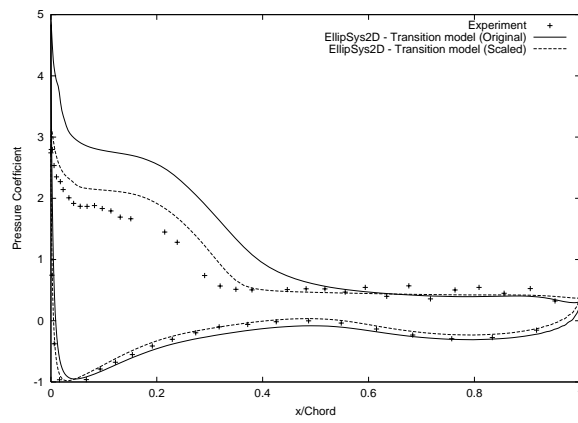
(d) Pressure Coefficient - \alpha = 15.11^\circ
