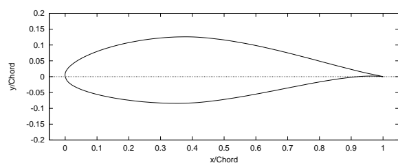
(e) NACA 64-421 Airfoil
