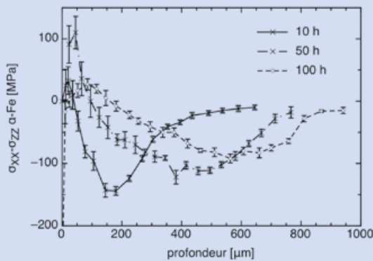
FIGURE 6 : Profils de contraintes résiduelles au sein de la ferrite de l'acier Fe-3% m .Cr-0.35% m .C nitruré à 550 °C pendant 10, 50 et 100 h. La contrainte moyenne \sigma_{xx}-\sigma_{zz} est obtenue par diffraction des rayons X et la méthode des \sin^2\psi .
