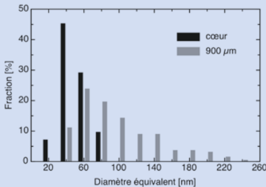
FIGURE 5 : Distribution en taille des précipités pour une profondeur de 900 μm (après 100 h de nitruration) et à cœur du matériau. Le nombre total de précipités pris en compte est de 188 et 236 respectivement.
