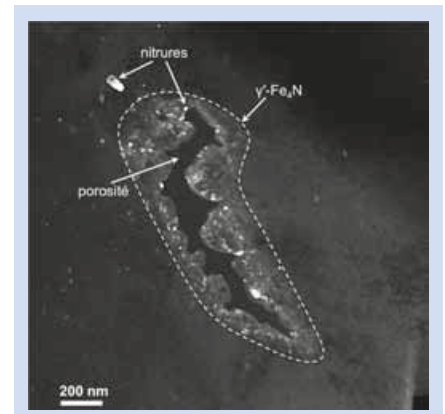
FIGURE 3 : Micrographie par microscopie électronique en transmission (en champ sombre) à 50 \mu\text{m} de profondeur de l'acier Fe-3% m.Cr-0.35% m.C nitruré à 550 °C pendant 100 h. Champ sombre à partir de l'intensité diffractée par les nitrures d'éléments d'alliage.
