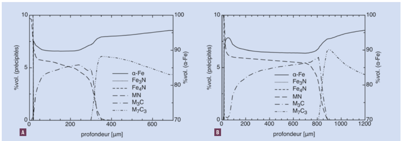
FIGURE 7 : Evolution de la fraction de phases à l'équilibre thermodynamique de l'acier Fe-3%Cr-0.35%MnC nitruré à 550 °C pendant (a) 10 et (b) 100 h. Les résultats sont calculés à partir de Thermo-Calc et des profils de composition chimique de la Figure 4.
