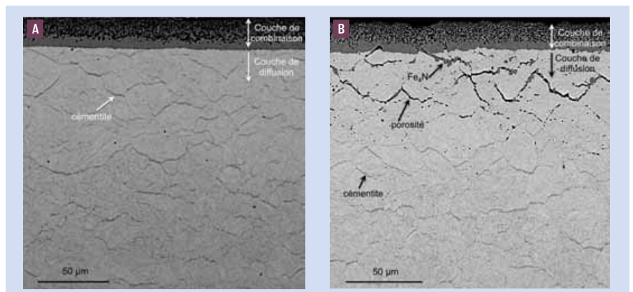
FIGURE 2 : Micrographies par microscopie électronique à balayage (image en électrons rétrodiffusés) de l'acier Fe-3%Cr-0.35%N nitruré à 550 °C pendant (a) 10 et (b) 100 h. Aucune attaque chimique préalable.
