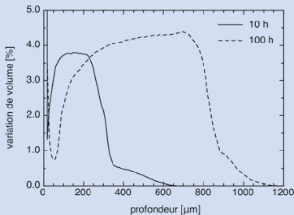
FIGURE 10 : Variations de volume calculées accompagnant la précipitation de l'acier Fe-3%Cr-0.35%Mn nitruré à 550 °C pendant 10 et 100 h. La transformation des carbures n'est pas prise en compte.
